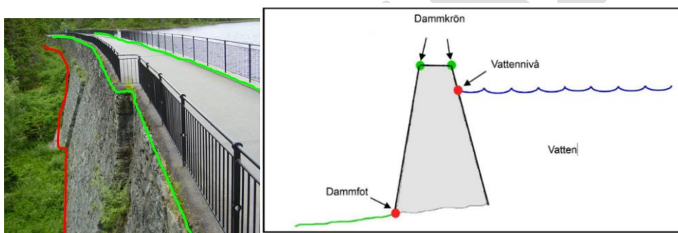
Figur D.2.1c. Dammbyggnad mäts med dammkrön (grön linje) samt dammfot (röd linje) och aktuell vattennivå (röd linje).
