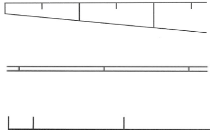
Figur 3.4.b. Kartbeteckningar för slänt, mur respektive stödmur. Slänt och stödmurs högsta kant markeras med korta streck Referens [5] .
