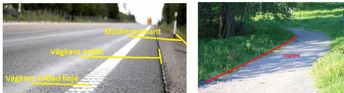
Figur 4.4a För HMK-standardnivå 2 redovisas vägar och gator med kantlinjer och marklinjen/transportlinjen kodas som vägbana. Kantlinjen för vägbana beskrivs av vägbana kantlinje (vänstra bilden) alternativt av tolkad vägbana för grusvägar (högra bilden), se även figur 4.4b.
