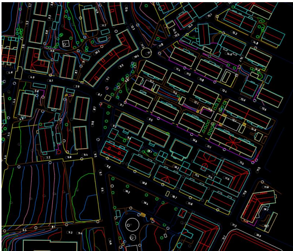
Figur 11c Utdrag ur kommunal geodatabas, dvs geodata i HMK-standardnivå 2, med redovisning i 2D. Om data lagras med höjder på redovisningslägena och höjdattribut-kan (Figur 11d) kan 3D-modeller tas fram vid behov.
