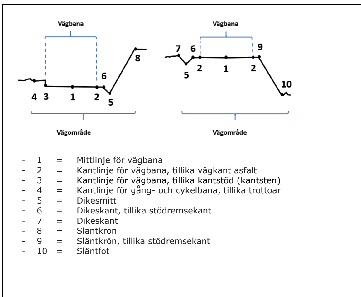
Figur 4.4b. Figuren avser tvärsektioner för väg med och utan gång- och cykelbana, se även figur 4.4a. Vägområde utgörs av den mark eller det utrymme som tagits i anspråk för väganordning och fastställs i vägplanen enl. väglagen – om sådan plan finns.
