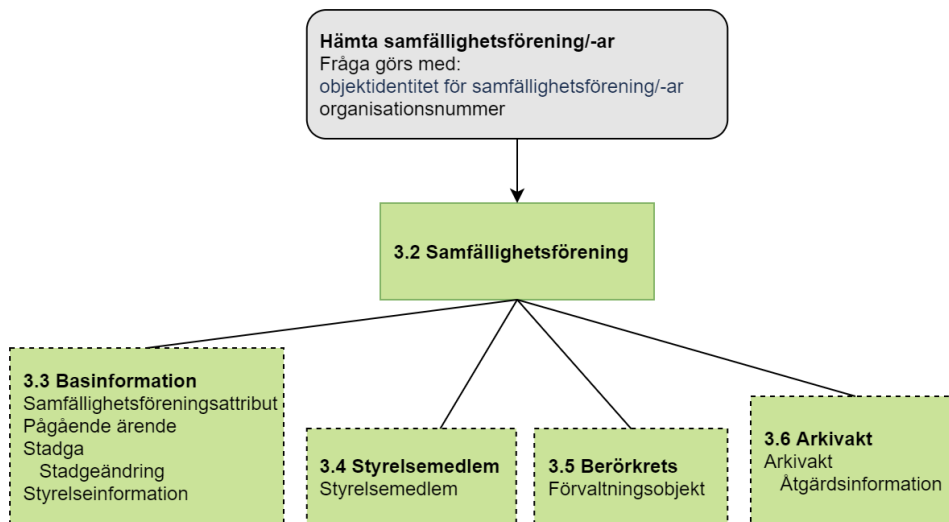
Figur 2. Beskrivning av frågan Hämta samfällighetsförening.
