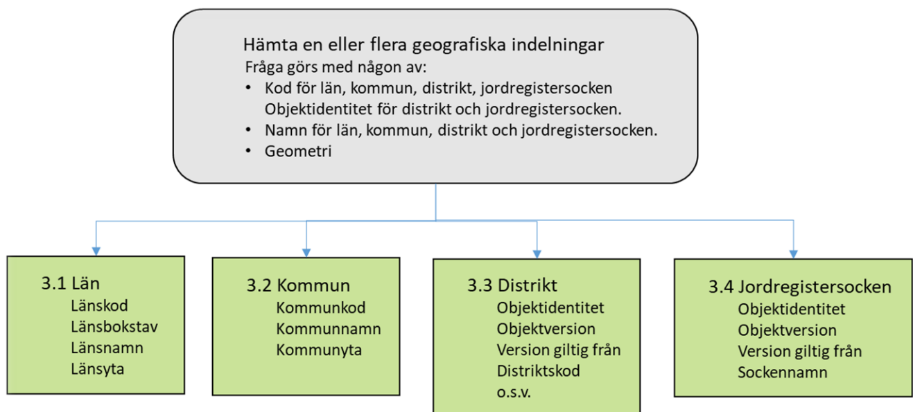
Figur 1. Illustration om hur informationen hänger ihop, hur frågor ställs och vilken information som ges i svaret.
