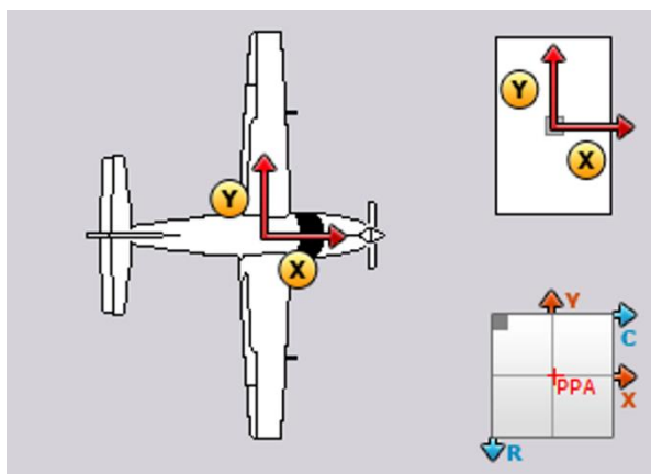
Figur 1. Om bildens centrum inte stämmer överens med kameranlinsens centrum används tabellen ovan för beräkning.
