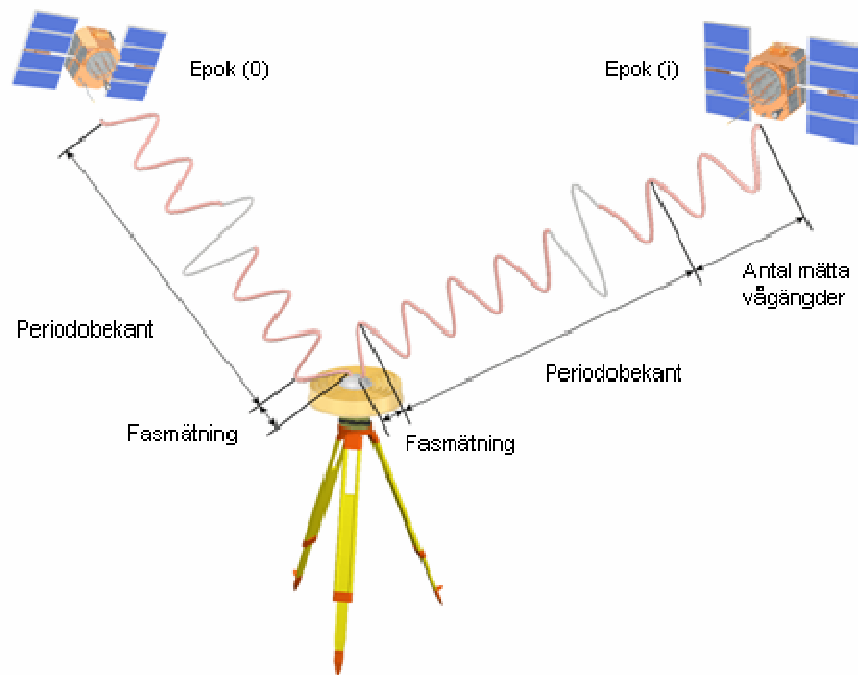
Figur 3: Bärvågsmätning.
