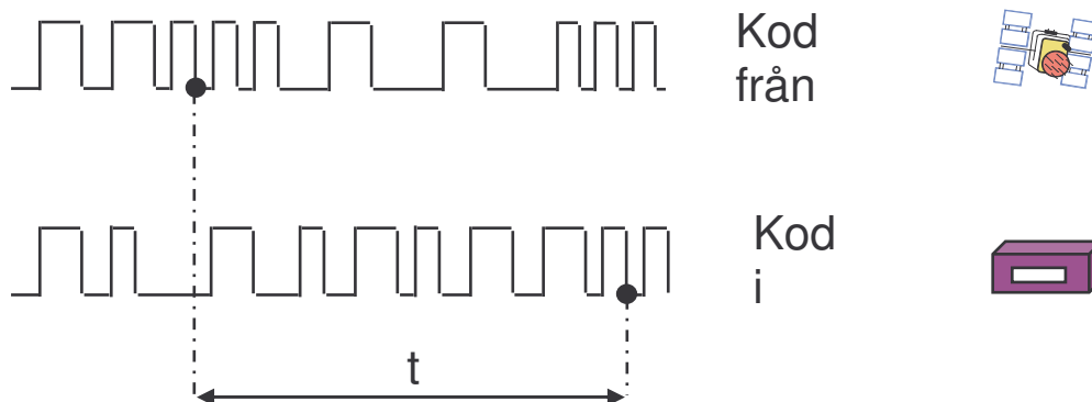
Figur 2: Kodmätning.
